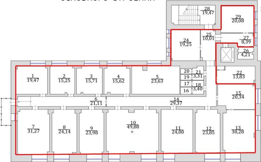
ПЛАН 3 ЭТАЖА ОСНОВНОГО СТРОЕНИЯ
